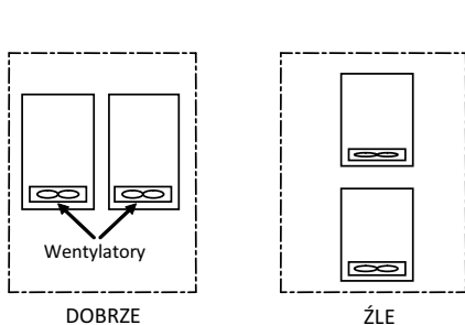
Umieszczenie kilku falowników w szafie
