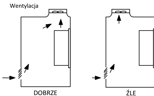
Instalacja wentylatora szafowego
